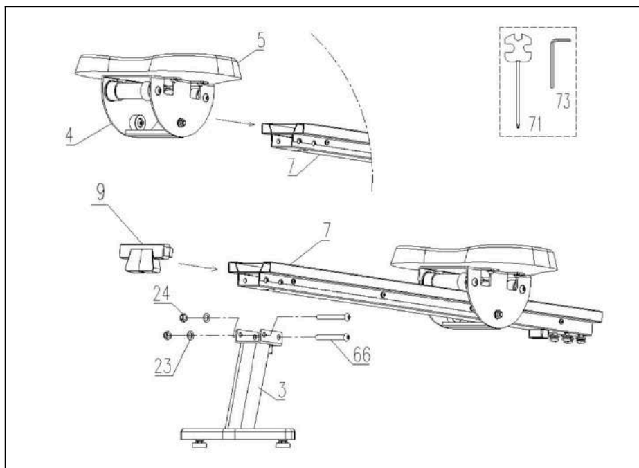
Рисунок 4 – Сборка направляющей
