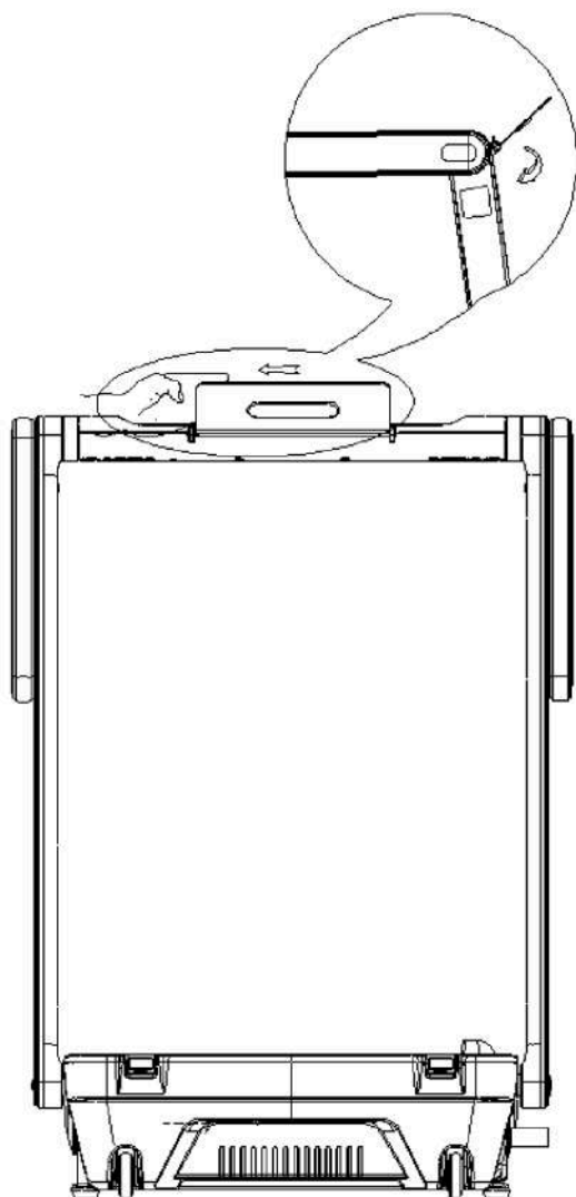
Рисунок 6 – Складывание подставки для гаджетов
