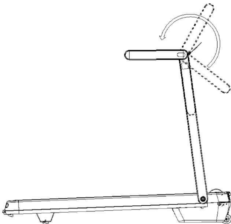
Рисунок 3 — Фиксация поручней
