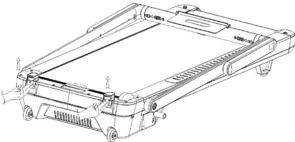
Рисунок 8 – Установка опорного ролика для транспортировки
