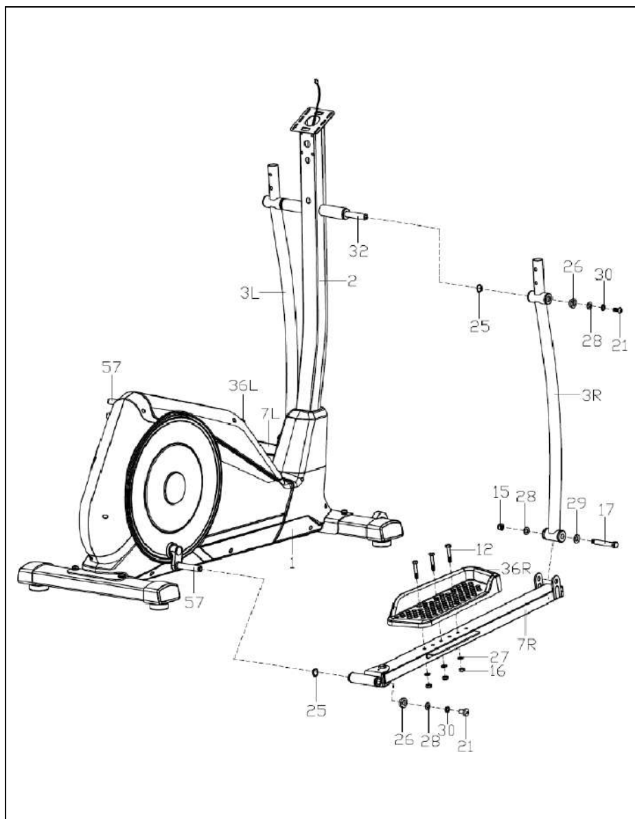
Рисунок 4 – Установка педалей
